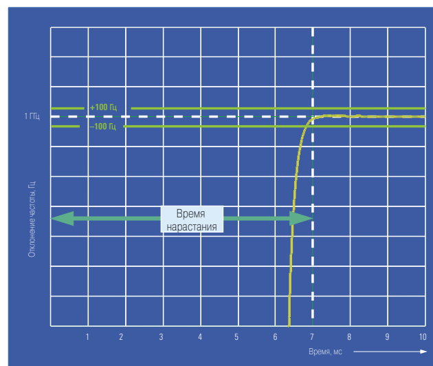
Свиппинг по уровню с диапазоном 25 дБ
