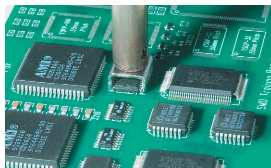
Демонтаж SOIC
